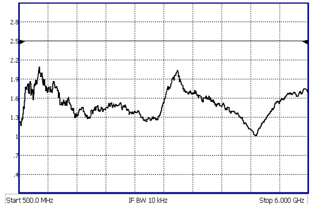
VSWR:
